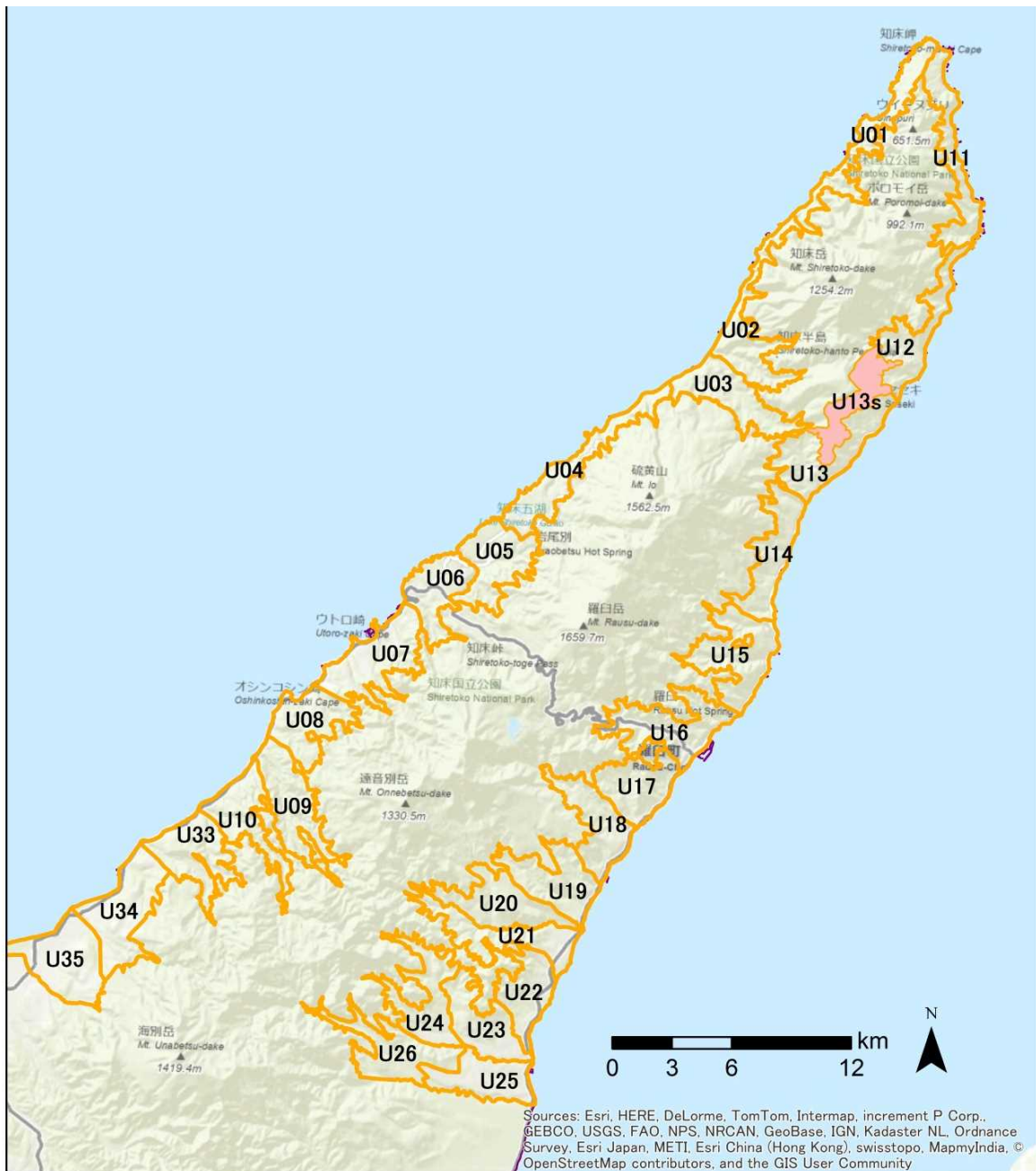
図：H27 シカ年度エゾシカ広域ヘリコプターカウント調査位置図 白抜きが標高 300m の標準調査区、塗りつぶしが標高 300～500m の高標高調査区（区域名の末尾に s）
